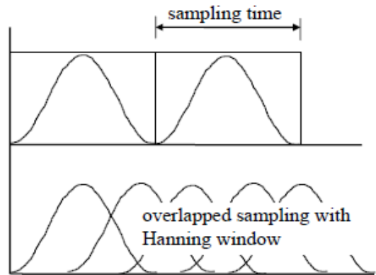
图16. 叠加采样
