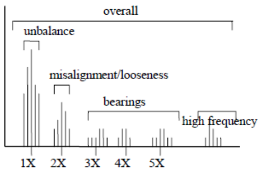
图20. 频带
