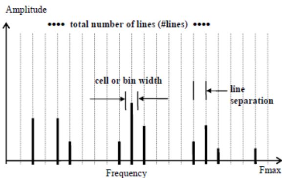
图8. FFT分辨率
